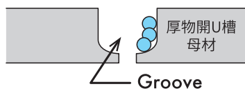
開槽時 (三)
